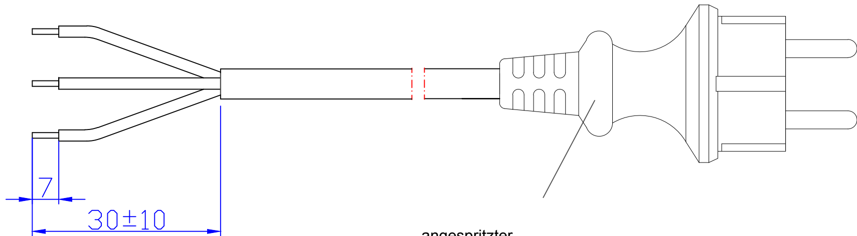
angespritzter Schutzkontakt-Zentralstecker Typ32
