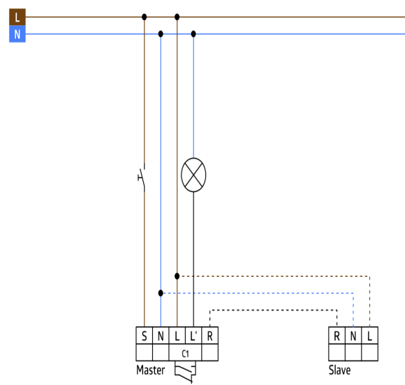
Schaltbild
