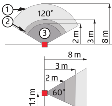
Reichweitendiagramm
