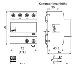
Maßbild DVA EMOB 3P 255 FM
