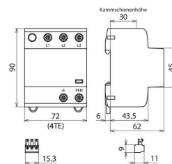
Maßbild DSH TNC 255 FM
