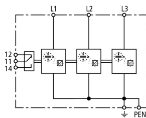
Prinzipialschaltbild DSH TNC 255 FM
