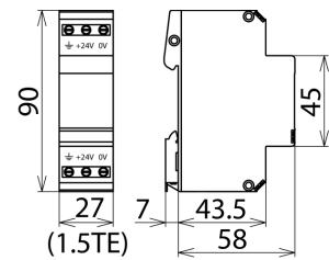
Maßbild BVT AVD
