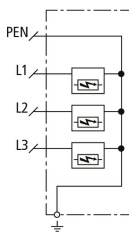
Prinzipschaltbild DSH ZP B2 TNC 255
