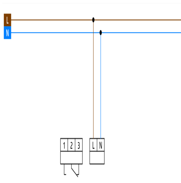
Schaltbild
