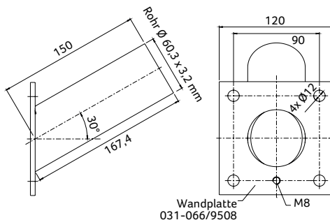
Abmessungen 30° Wandhalterung (Art.-Nr. 18953)
