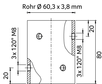
Abmessungen Adapter (Art.-Nr. 18955)
