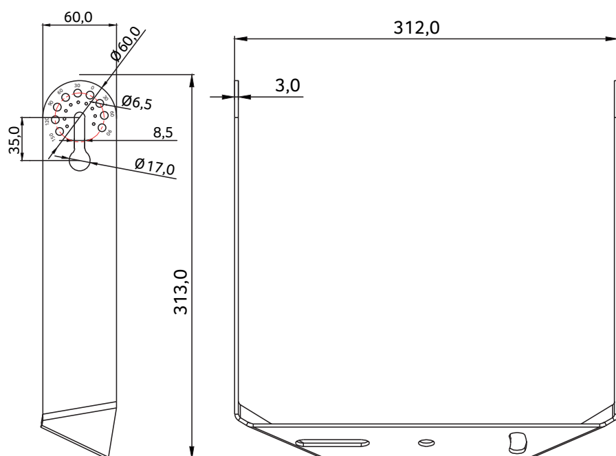
Abmessungen Wandmontagebügel 100 / 150 / 200 Watt (Art.-Nr. 18965)
