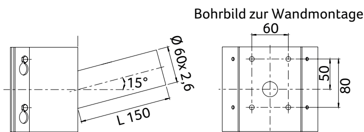
Abmessungen Wand-Eckhalter (Art.-Nr. 18958)
