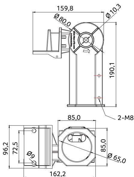
Abmessungen Adapter für Mastansatz- und Mastaufsatzmontage (Art.-Nr. 18963)
