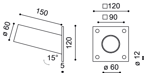
Abmessungen 15° Wandhalterung (Art.-Nr. 18954/18959)
