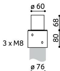
Abmessungen Adapter (Art.-Nr. 18956)
