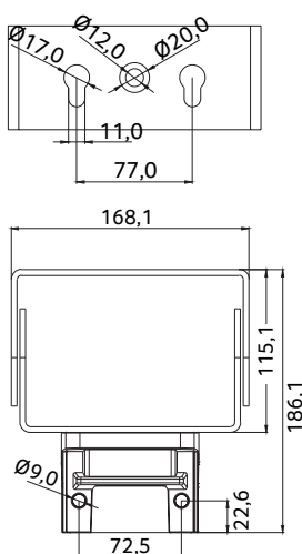
Abmessungen Adapter für Wandmontage (Art.-Nr. 18964)
