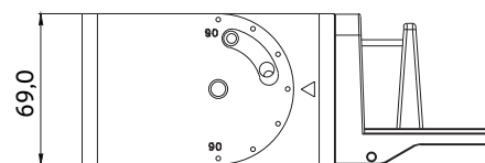
Einstellmöglichkeiten Adapter für Wandmontage (Art.-Nr. 18964)
