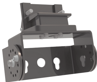
Adapter für Wandmontage (Art.-Nr. 18964)
