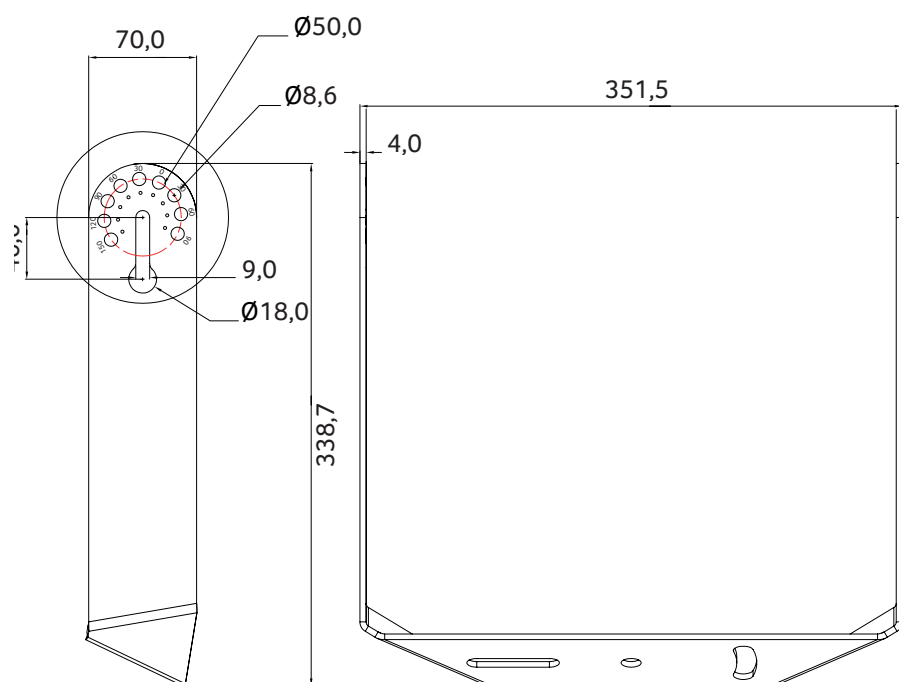
Abmessungen Wandmontagebügel 400 Watt (Art.-Nr. 18971)
