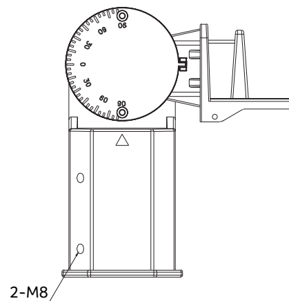
Einstellmöglichkeiten Adapter für Mastansatz- und Mastaufsatzmontage (Art.-Nr. 18963)
