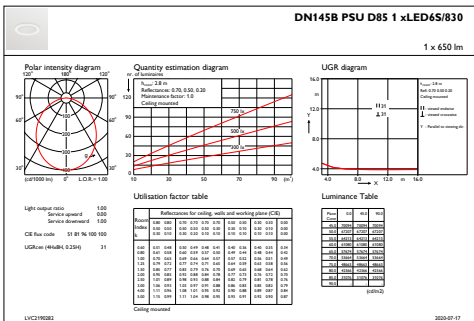
IFGU1_DN145BPSUD851xLED6S830
