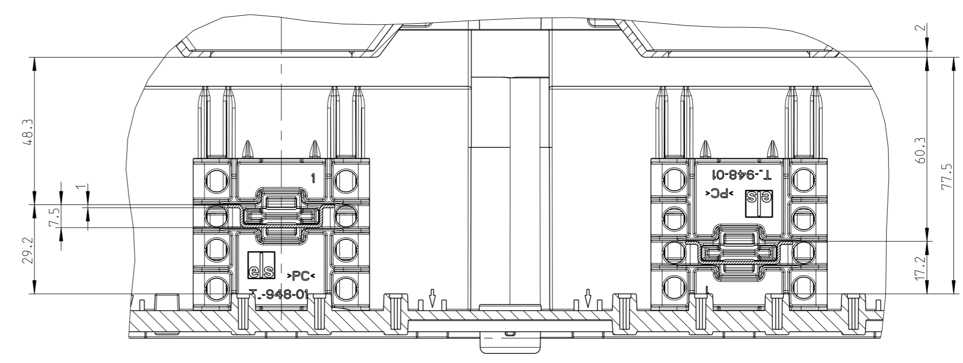
A-A Detail um 90° gedreht 4:5
