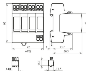
Maßbild DG MP TT 275 FM
