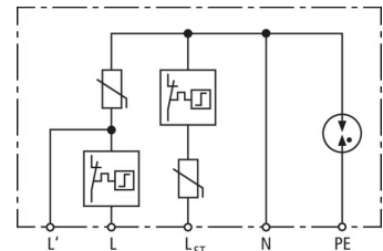
Prinzipschaltbild DEHNcord
