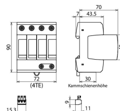
Maßbild DG M TT ACI 275 FM
