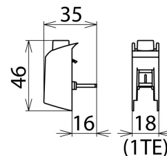
Maßbild STAK 25
