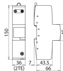
Maßbild DVCI 1 255
