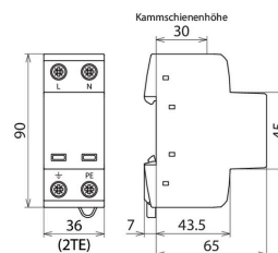
Maßbild DSH TT 2P 255
