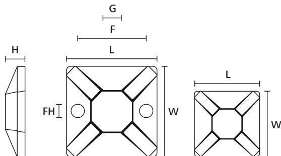
MB3-MB5 (Seitenansicht)
