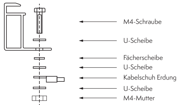
empfohlene Montageart für den Erdungsanschluss
