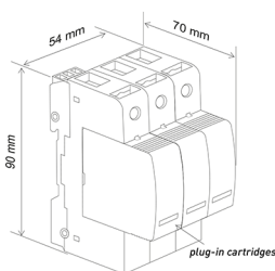
Dreipolig
