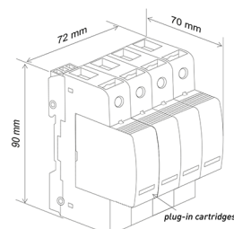
Vierpolig
