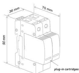
Zweipolig
