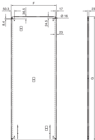
Montageplatte
