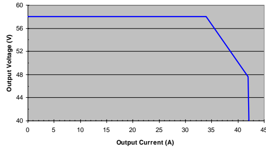
Ausgangsspannung zu Ausgangsstrom (AC In = 185V, Vaus = 48.0V)
