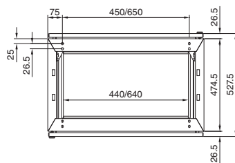
Montageplatte
