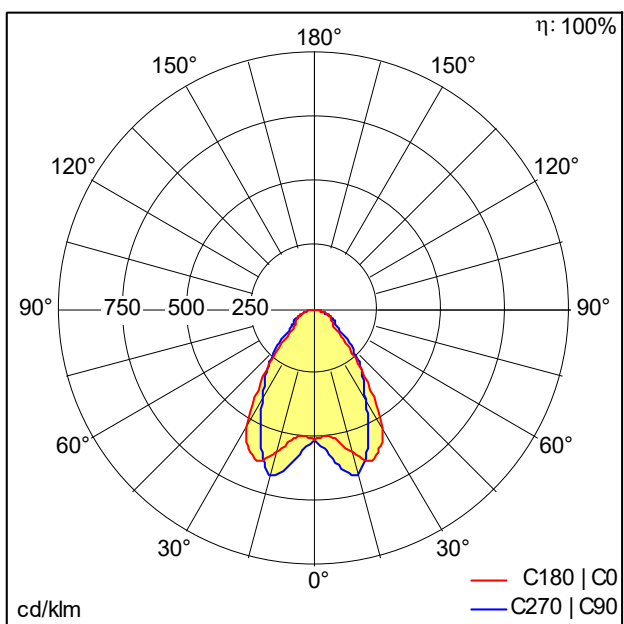
TECTON_C_10000_840_L2000_WB_LDE_WH.Idt
