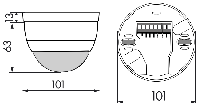
Bemaßung 92440
