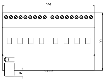
Bemaßung 93339
