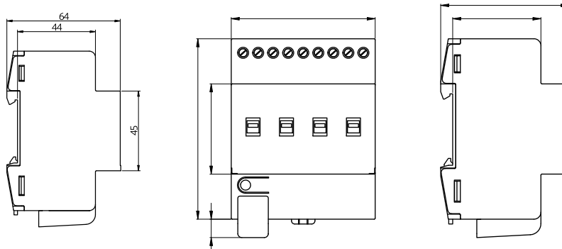
Bemaßung 90136
