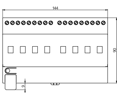
Bemaßung 93336
