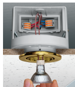
Individueller Aufbau von Niedervolt-Beleuchtungssystemen
