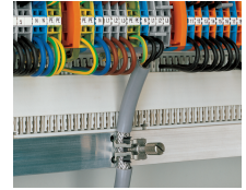
Schirmklemmbügel auf Befestigungsblechen bis 3 mm Dicke
