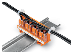
Zugentlastung durch Kabelbinder am Adapter, quer zur Klemmenanschlussrichtung; Klemmstellenkennzeichnung durch Beschriftungsstreifen (210-334)
