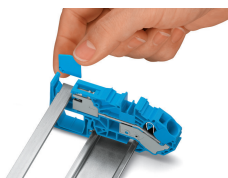
Einsetzen der herausgebrochenen Trennplatte in die N-Trennklemme
