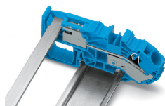
Mittels eingesetzter Trennwand entsteht eine berührungsgeschützte N-Sammelschiene.
