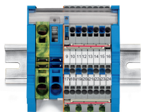
Sammelschienen sind in Sammel-schienen-trägern zu montieren. Dabei sind Sammel-schienenenden in breiten Trägern (Bestellnr. 2009-305) oder in Einspeiseklemmen mit integriertem Sammel-schienen-träger einzurasen.
