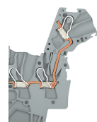
L-Prüfsteckmodul, Kontaktierungsschnittbild
