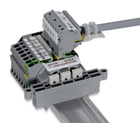
Motoranschluss-Klemmenblock
