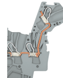
L-Prüfsteckmodul, Kontaktierungsschnittbild
