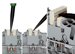
Kammbrücker lösen Mit dem Betätigungswerkzeug zwischen Brücke und Trennsteg der Brückerschächte eintauchen und Brücke heraushebeln. Bei Brückern (5-fach) Betätigungswerkzeug mittig ansetzen (siehe Abb. 3), ab 5-fach wechselseitig.
