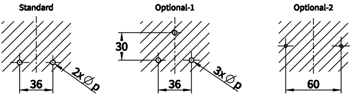
Montageausschnitt/ Mounting cutout
