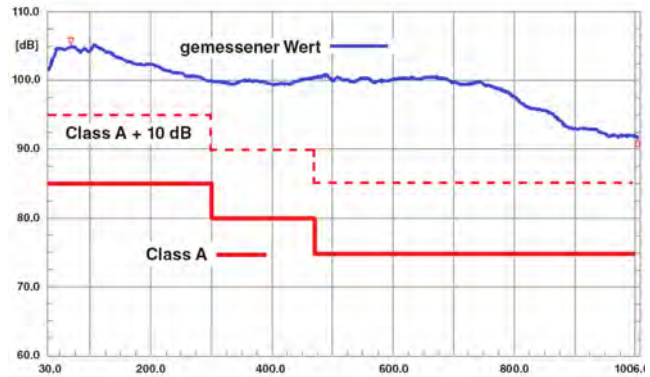
EMV Messung am neuen GUT-Anschlussdosenchassis
