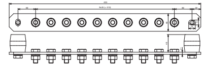
Maßbild
