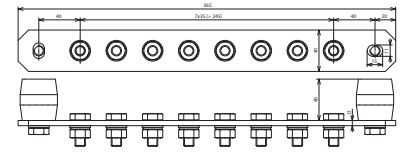
Maßbild
