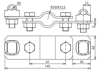
Maßbild
