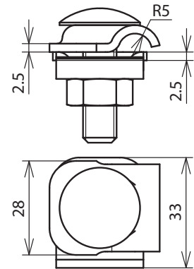
Maßbild
