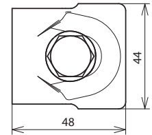
Maßbild
