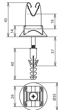
Maßbild
