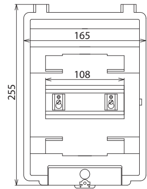
Maßbild
