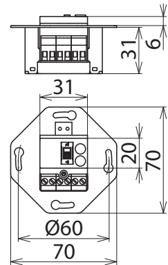
Maßbild
