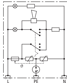
Prinzip Schaltbild
