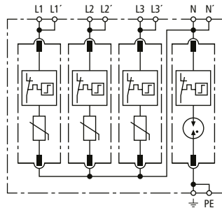
Prinzipschaltbild
