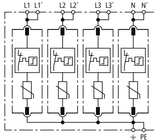
Prinzipschaltbild
