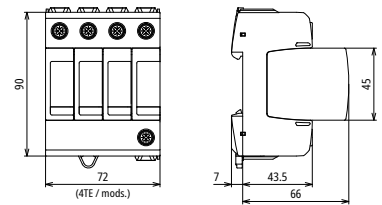
Maßbild
