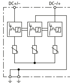
Prinzipschaltbild
