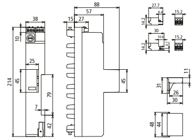
Maßbild
