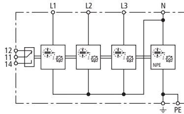
Prinzipschaltbild
