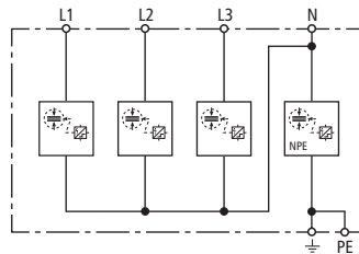
Prinzipschaltbild
